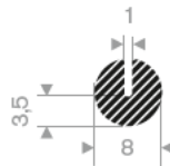
221.01.108 EPDM 15° Shore rollengte 100 meter
