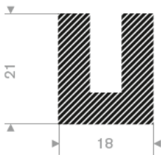
221.00.160 EPDM 15° Shore rollengte 50 meter
