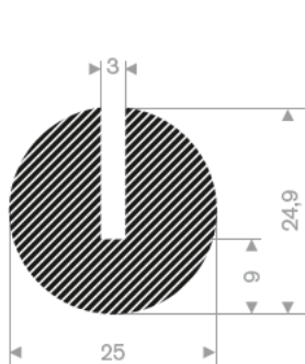
221.01.088 EPDM 15° Shore rollengte 25 meter
