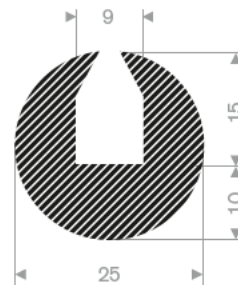
221.01.825 EPDM 15° Shore rollengte 30 meter
